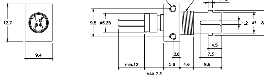
ST Receptacle
