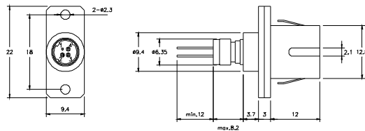
SC Receptacle
